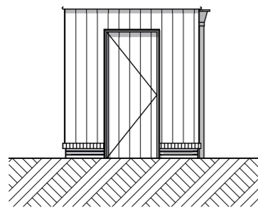
1:100 Voorgevel
