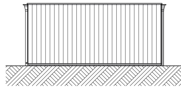
1:100 Achtergevel
