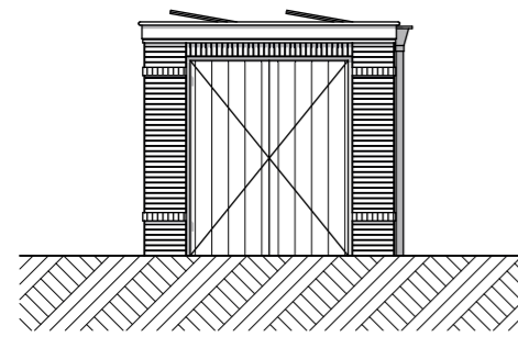
1:100 Voorgevel
