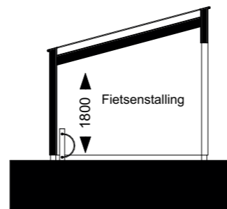
1:100 Doorsnede A-A
